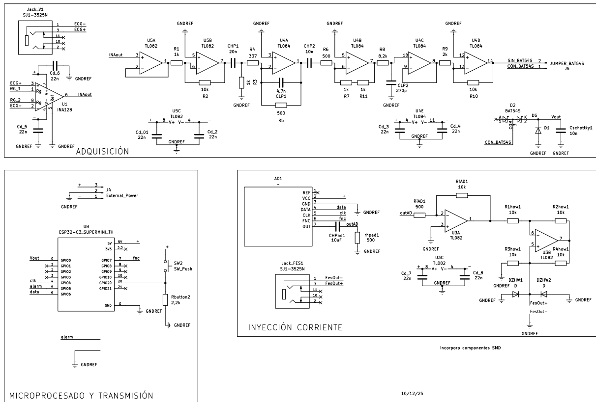
Figura 13: Esquema electrónico general. Los detalles del acondicionamiento se presentan ampliados en la sección de adquisición.
