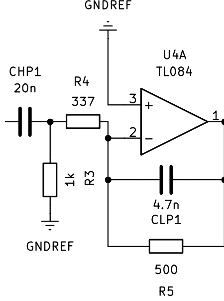
Figura 8: Primer acoplamiento pasaaltos y filtro inversor U4A.
