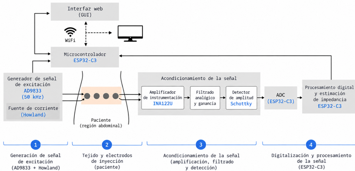
Figura 3: Diagrama de bloques del sistema de medición de bioimpedancia. El ESP32-C3 configura la excitación, digitaliza la señal detectada y transmite los resultados a la interfaz gráfica.
