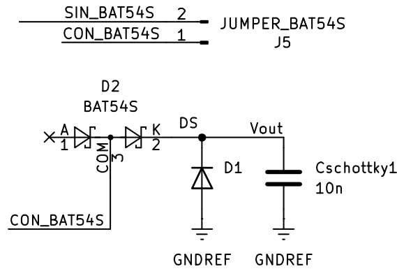
Figura 12: Conexiones de selección en J5 y bloque detector con salida Vout.
