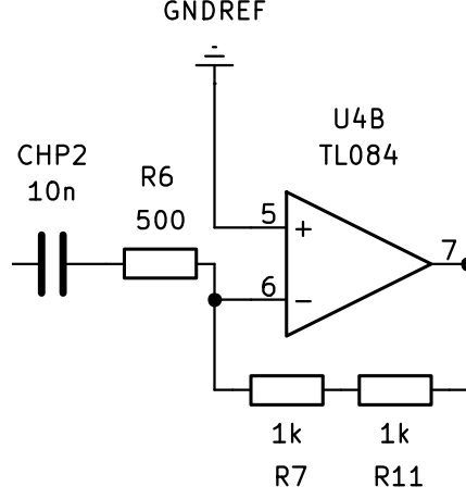
Figura 9: Segundo pasaaltos activo con U4B; R7 y R11 forman la realimentación.
