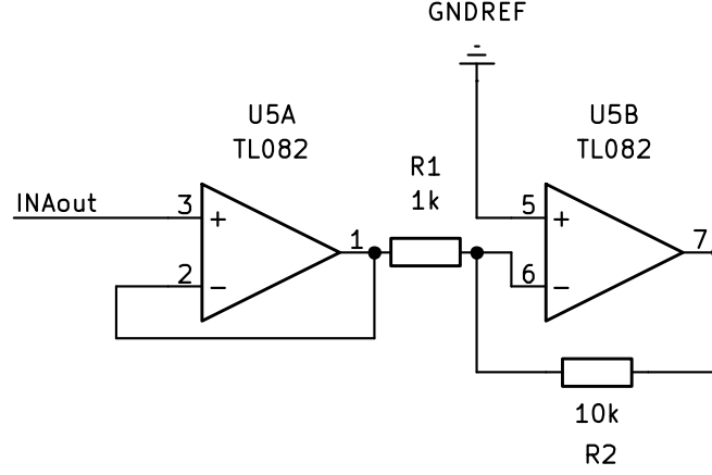
Figura 7: Seguidor U5A y amplificador inversor U5B, desde la entrada INAout.
