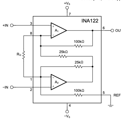
Figura 5: Estructura interna del INA122 y conexión de la resistencia externa de ganancia. En el diseño se dejan abiertos los terminales de dicha resistencia para obtener una ganancia nominal de 5. Esquema de Texas Instruments [25].
