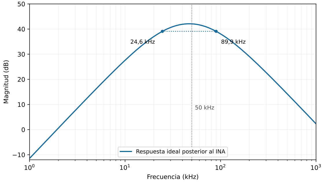
Figura 11: Diagrama de Bode de magnitud ideal de las seis etapas posteriores al INA, calculado como 20 \log_{10} |H_{ac}| . Se indican la frecuencia de excitación de 50 kHz y los límites de banda a aproximadamente -3 dB respecto del máximo. La curva corresponde al cálculo teórico, no a mediciones experimentales.
