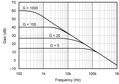
Figura 6: Respuesta en frecuencia del INA122 para distintos valores de ganancia. Para G = 5 , la frecuencia de corte se encuentra aproximadamente en 100 kHz, mientras que a 50 kHz la ganancia ya presenta una atenuación respecto de su valor de baja frecuencia. Adaptada de Texas Instruments [25].
